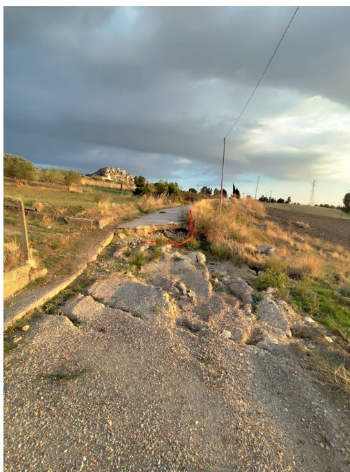
Foto 02 - Dissesto della carreggiata e tratto non percorribile
